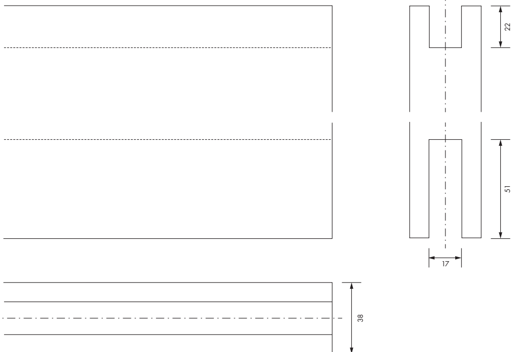
Dichtungsset horizontal
