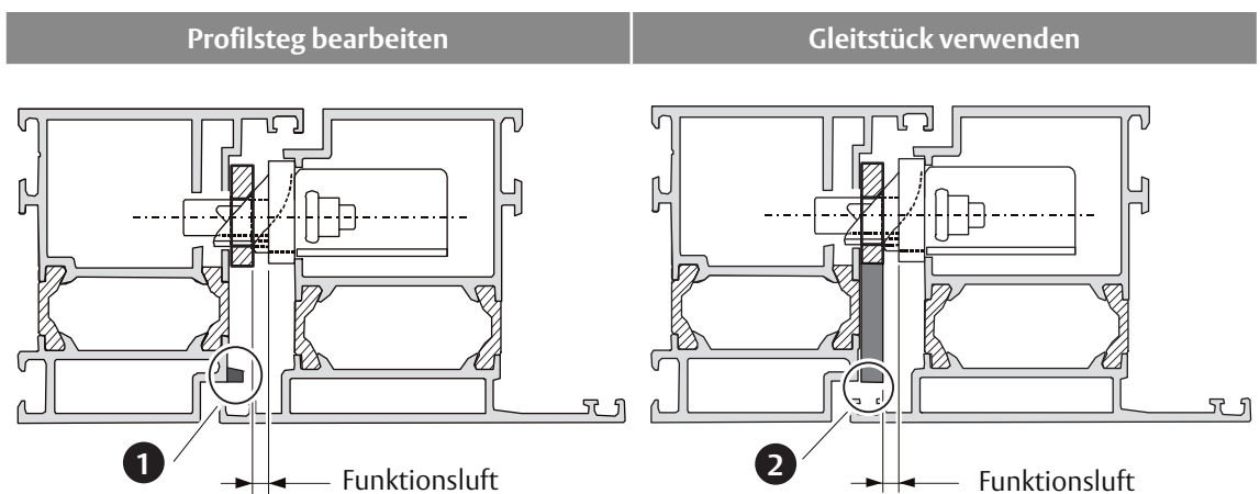
Abb. 16: Profilsteg nachbearbeiten und Gleitstück verwenden
