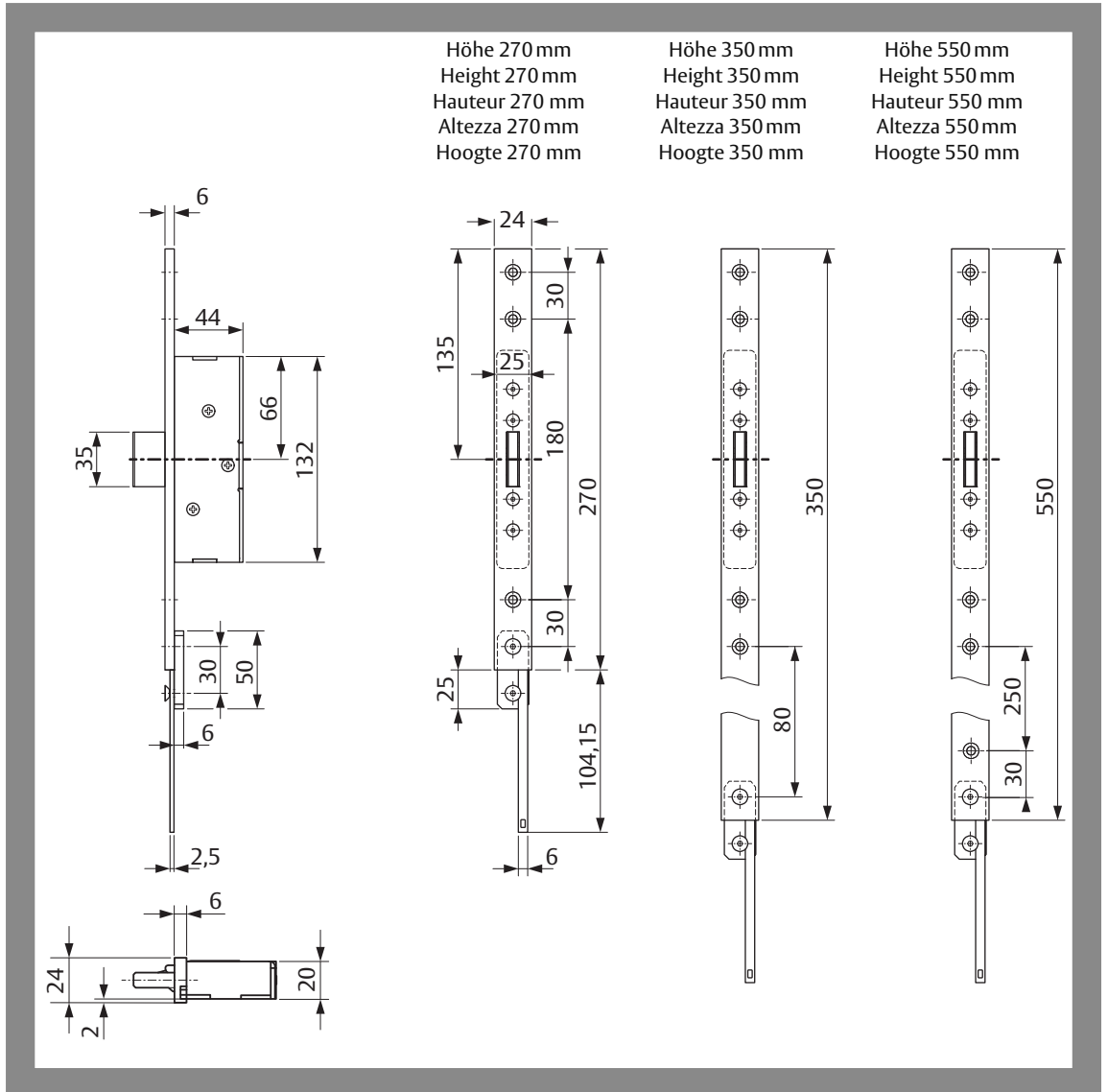
Abb. 25: Abmessungen Zusatzriegel
