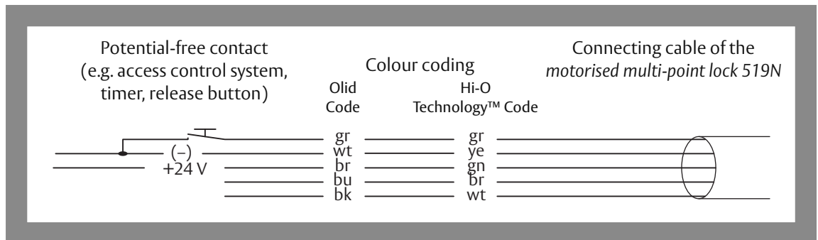
Fig. 15: Wiring diagram
