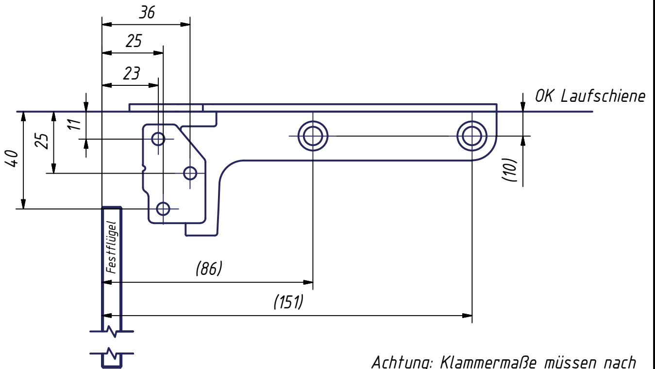
Lochbild ausziehbarer Spritzschutz, rechts
