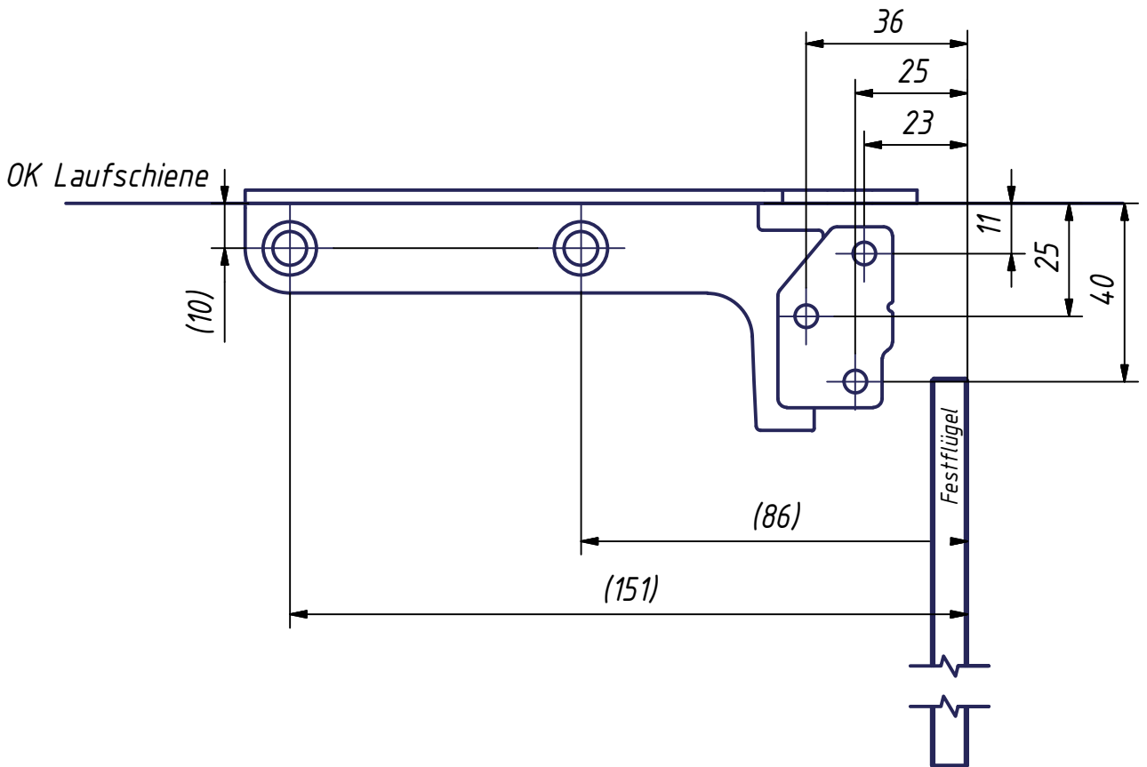
Lochbild ausziehbarer Spritzschutz, links
